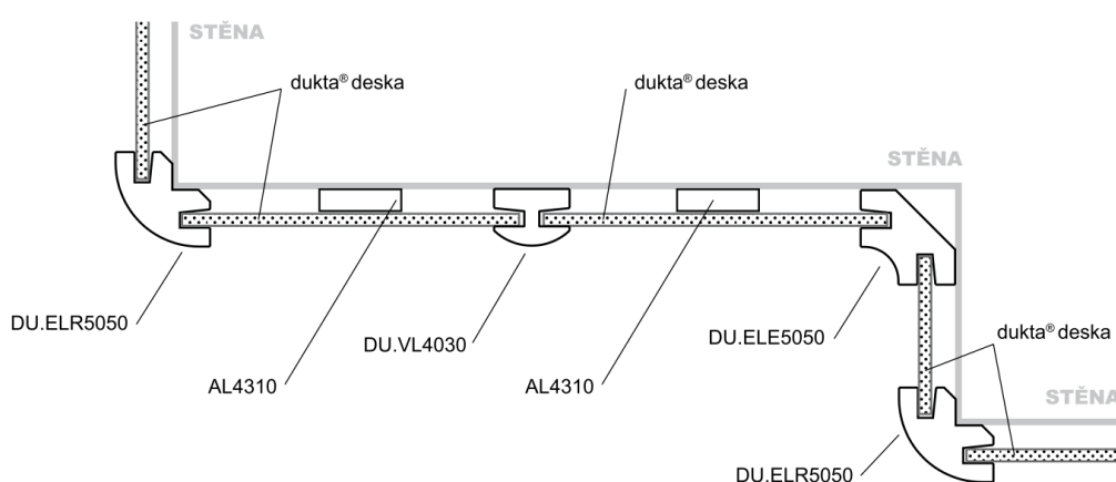
vnější roh
