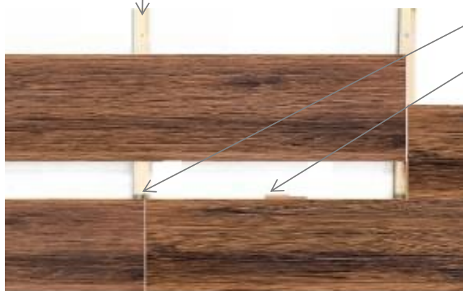
montážní lišta smrk 50 x 20 mm
